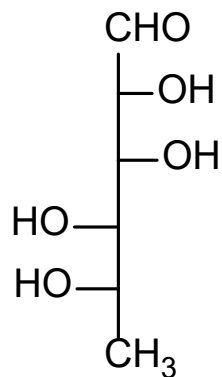
L-rhamnose
