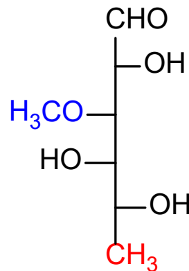
D-digitalose
