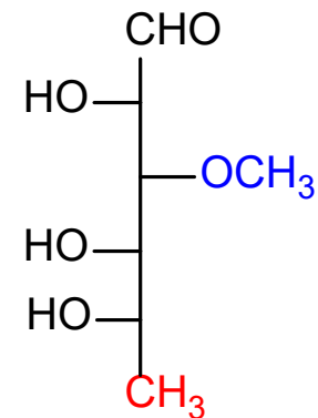
L-thevetose
